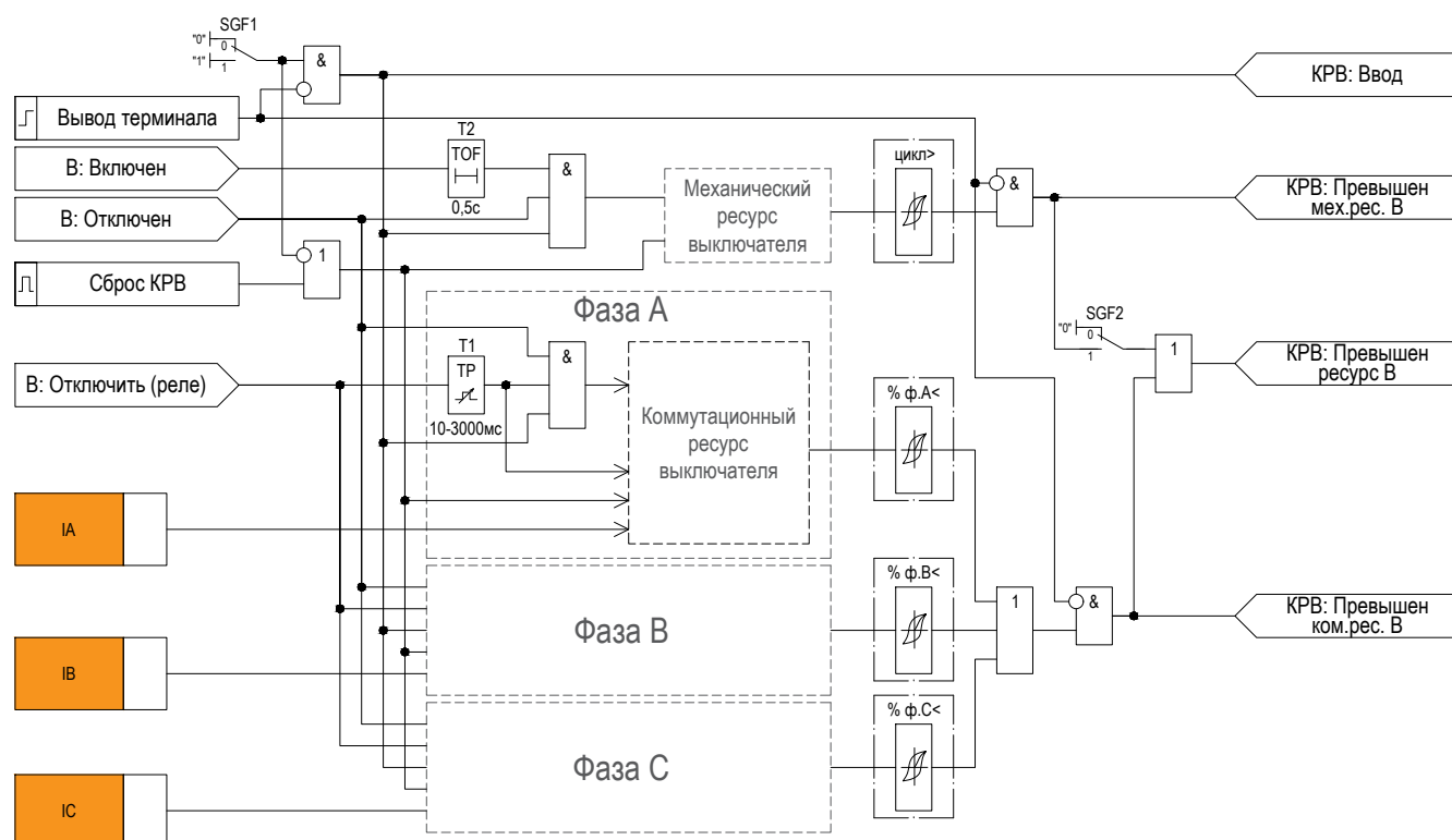
Рисунок 2.69 – Функциональная схема «КРВ»
