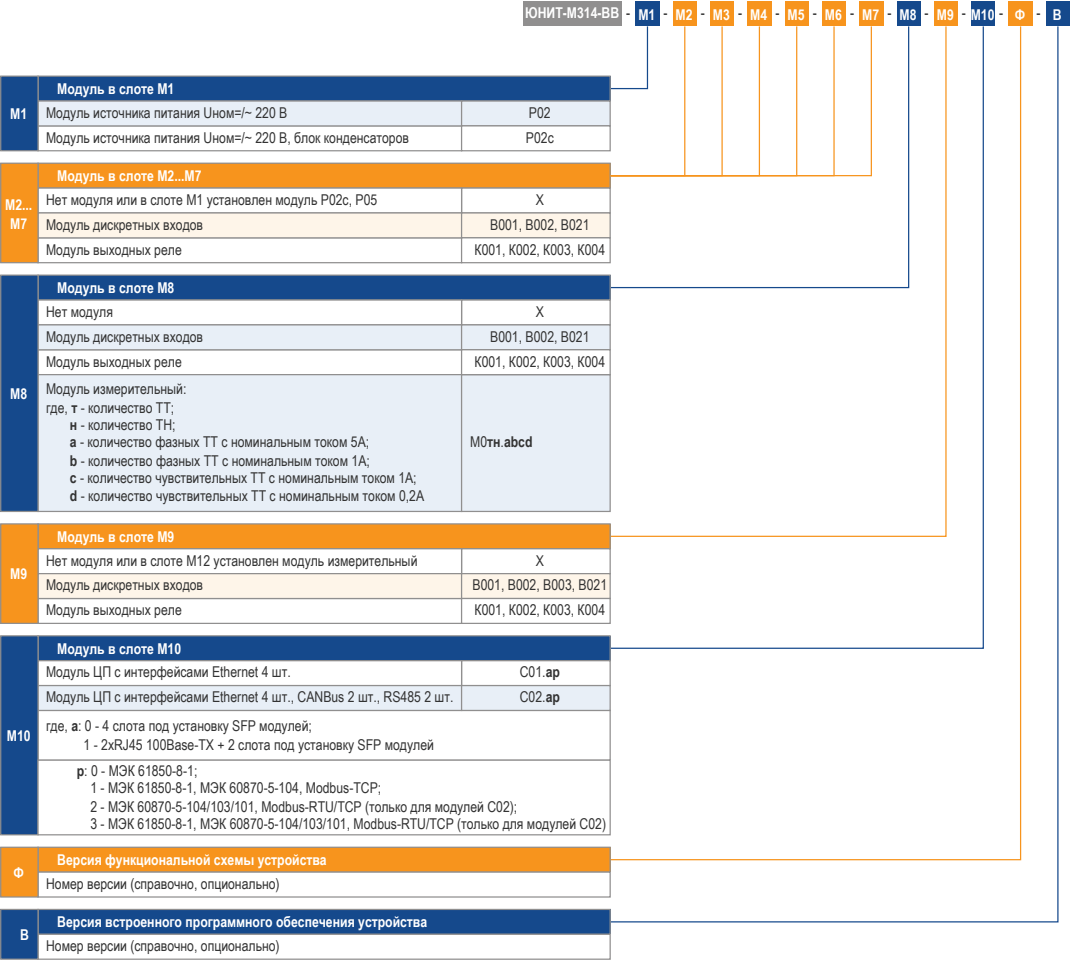
Рисунок А.1 – Код заказа устройства «ЮНИТ-М314-ВВ»
