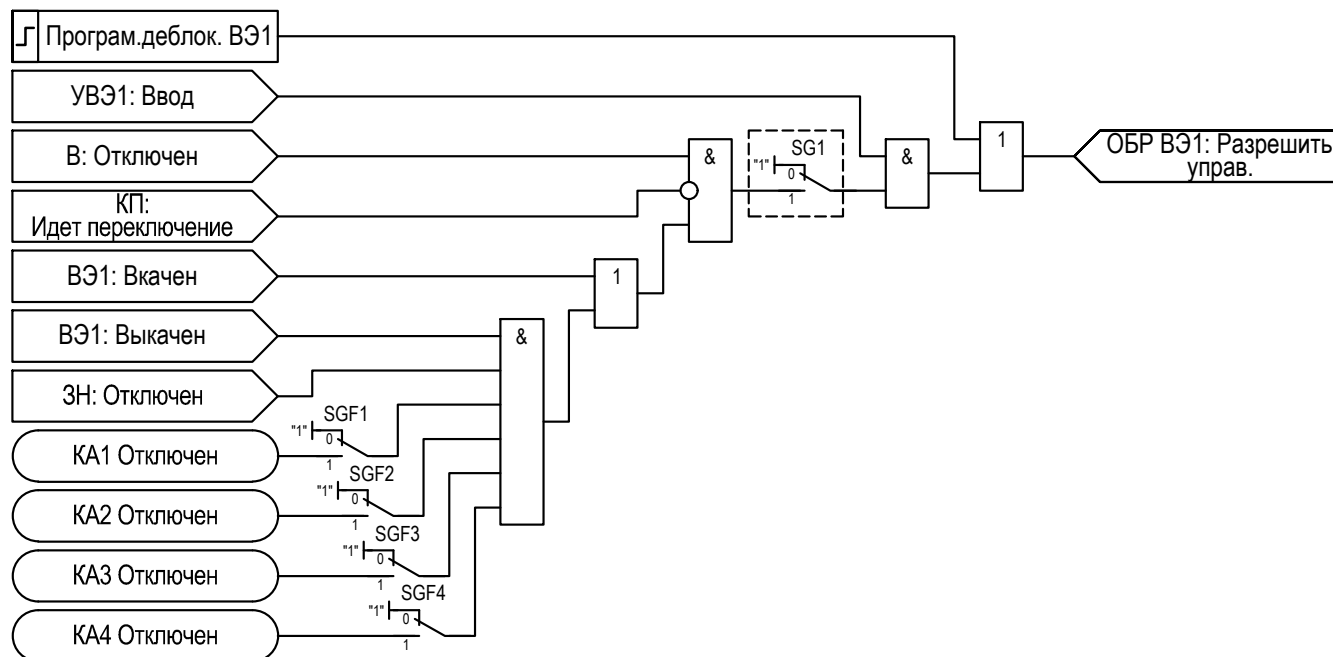
Рисунок 2.61 – Функциональная схема «ОБР ВЭ1»
