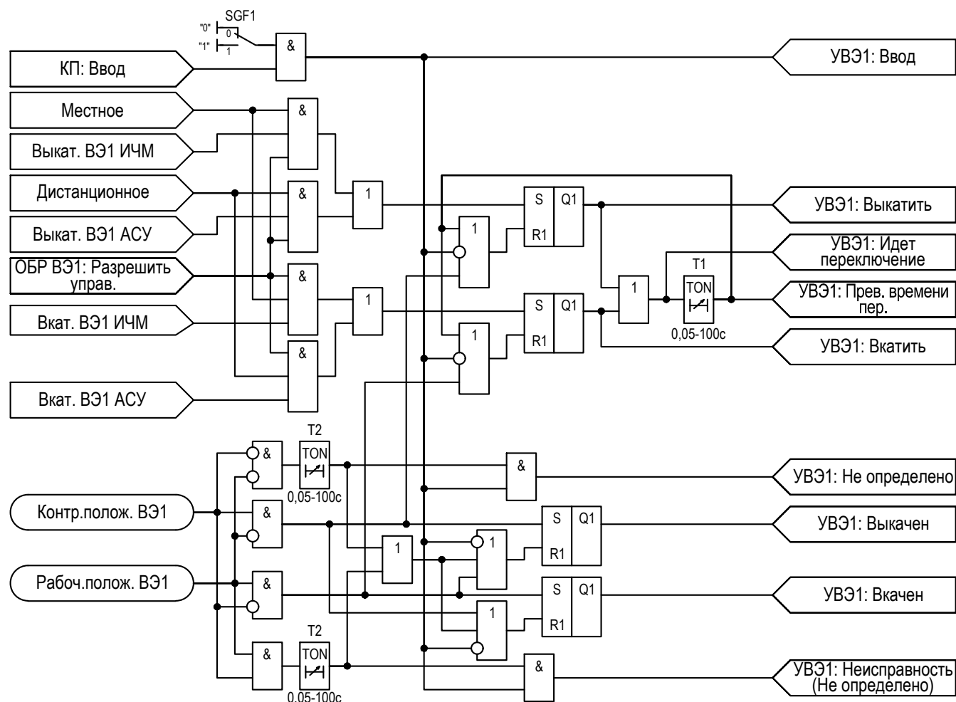
Рисунок 2.57 – Функциональная схема «УВЭ1»
