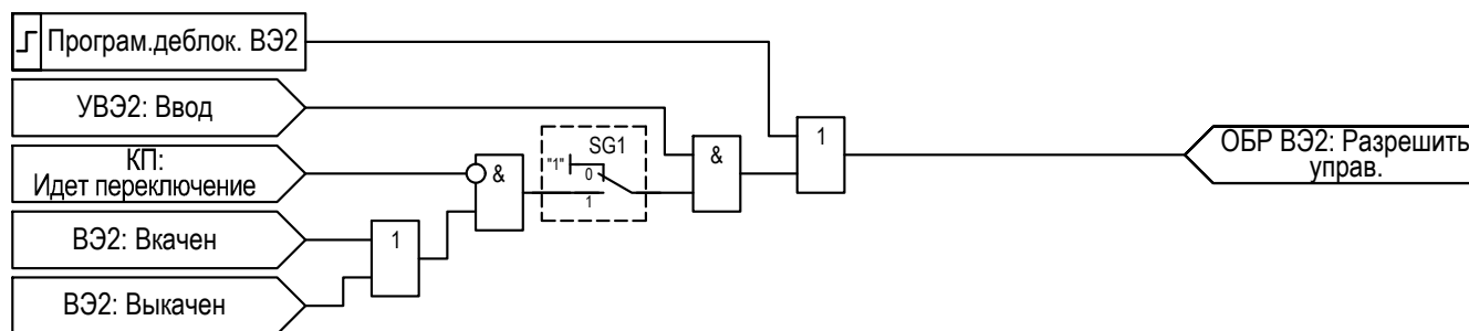
Рисунок 2.62 – Функциональная схема «ОБР ВЭ2»
