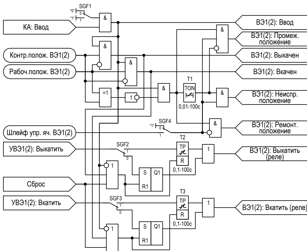
Рисунок 2.67 – Функциональная схема «ВЭ1(2)»
