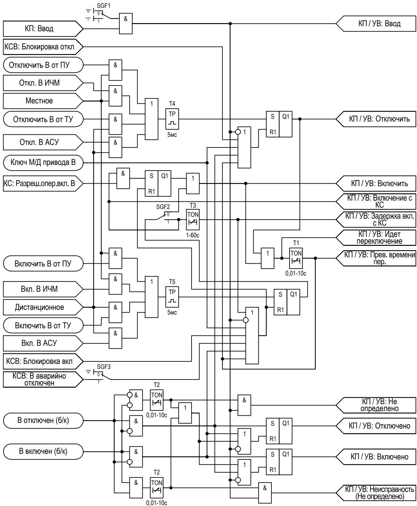
Рисунок 2.55 – Функциональная схема «УВ»
