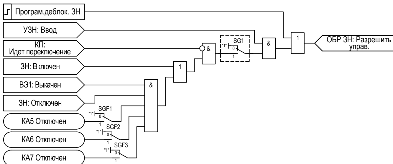
Рисунок 2.60 – Функциональная схема «ОБР 3Н»
