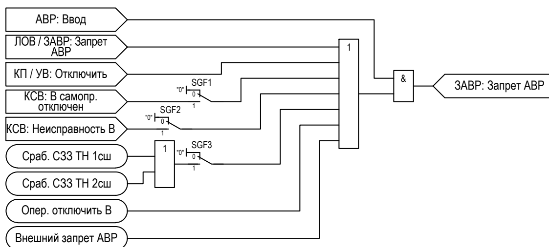
Рисунок 2.45 – Функциональная схема «ЗАBP»
