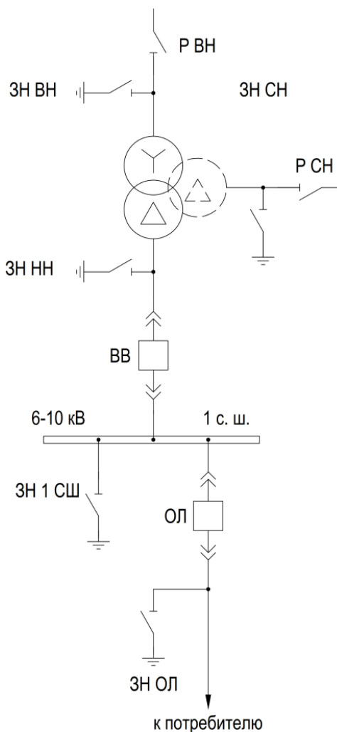
Рисунок 2.58 – Поясняющая схема первичной сети для алгоритмов оперативной блокировки КА
