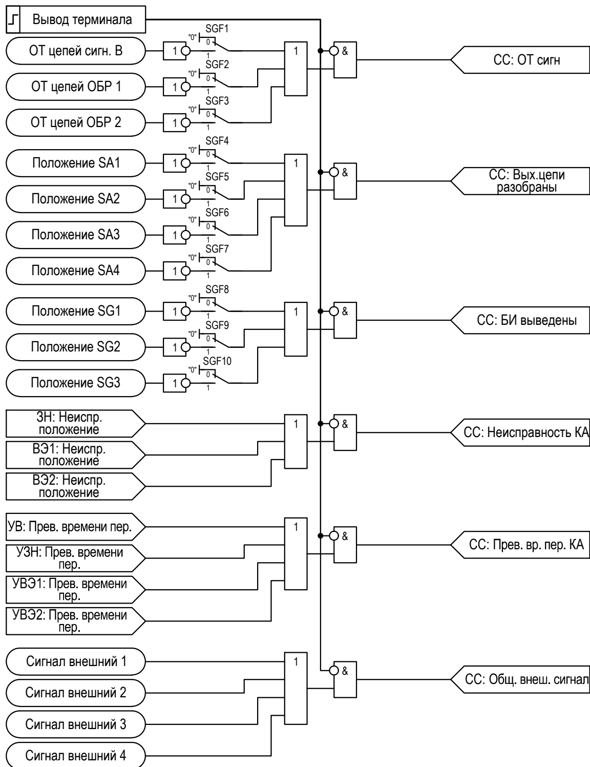
Рисунок 2.70 – Функциональная схема «СС»
