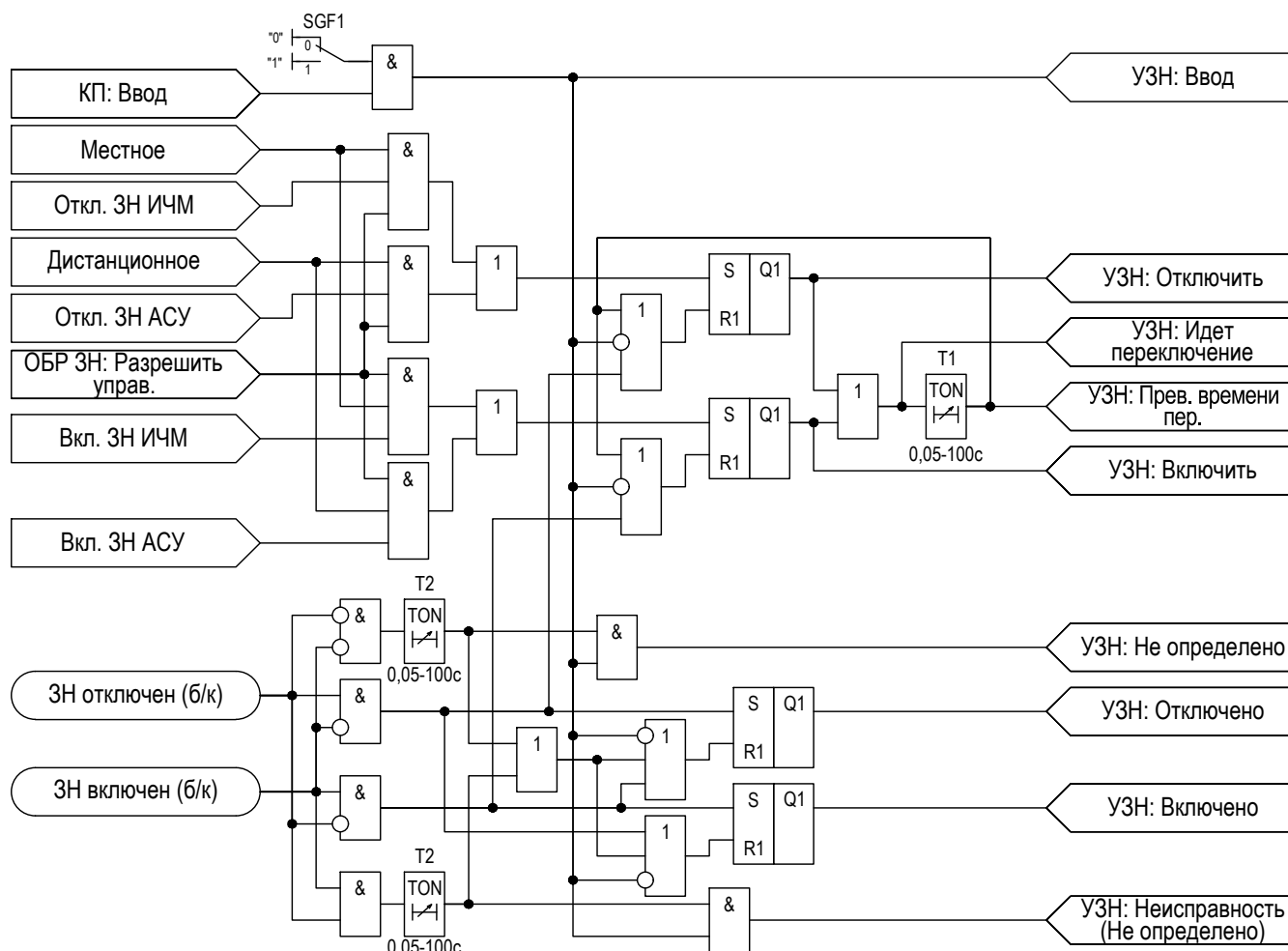
Рисунок 2.56 – Функциональная схема «УЗН»
