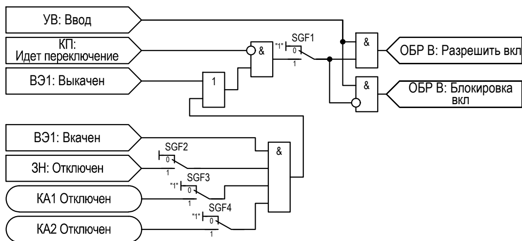
Рисунок 2.59 – Функциональная схема «ОБР В»
