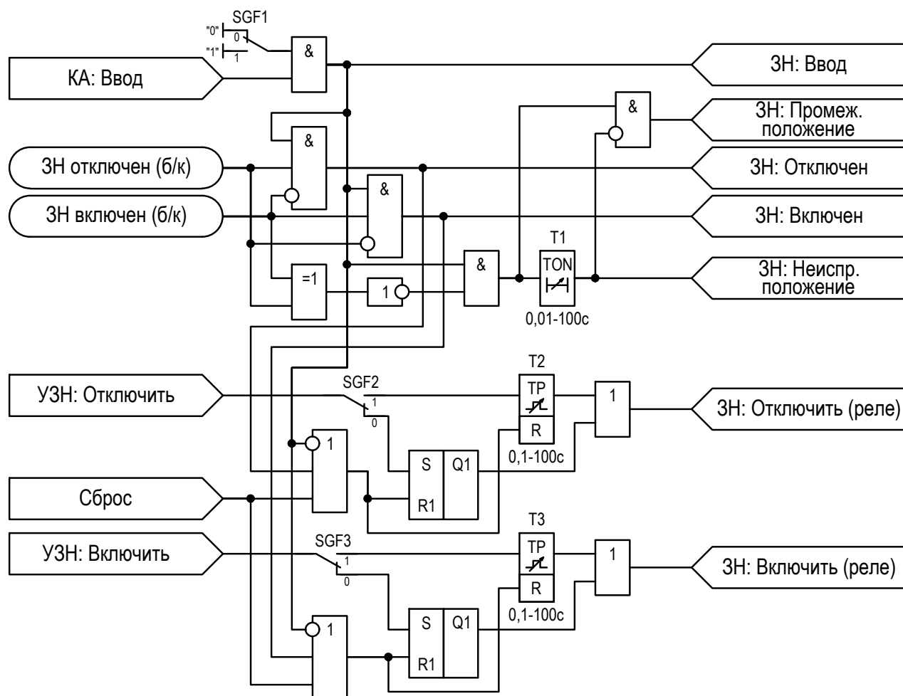
Рисунок 2.66 – Функциональная схема «ЗН»
