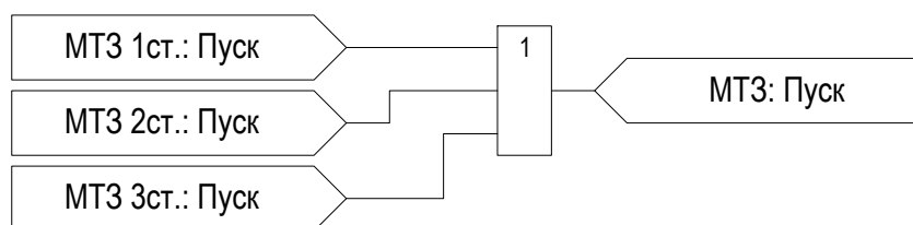
Рисунок 2.24 – Функциональная схема внешней логики МТЗ
