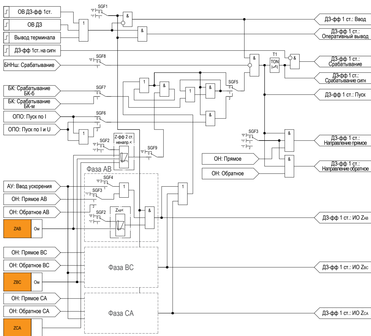
Рисунок 2.2 – Функциональная схема «ДЗ-фф 1ст.»
