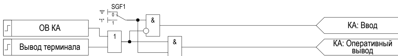
Рисунок 2.64 – Логика управления режимами функционального блока «КА»
