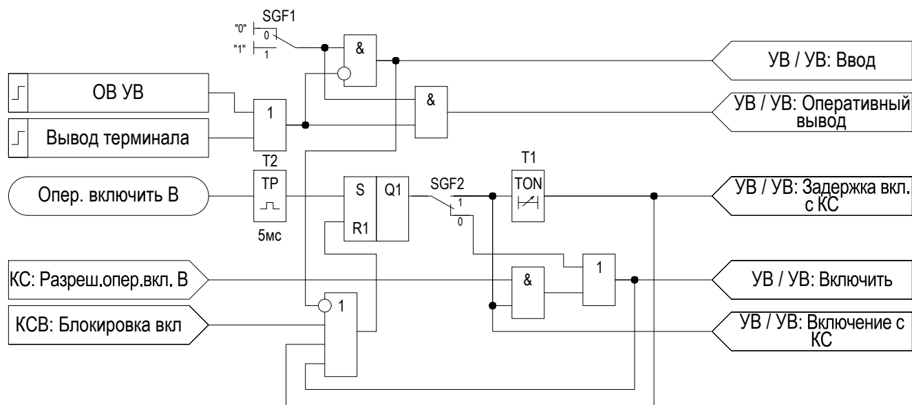
Рисунок 2.63 – Функциональная схема «УВ»
