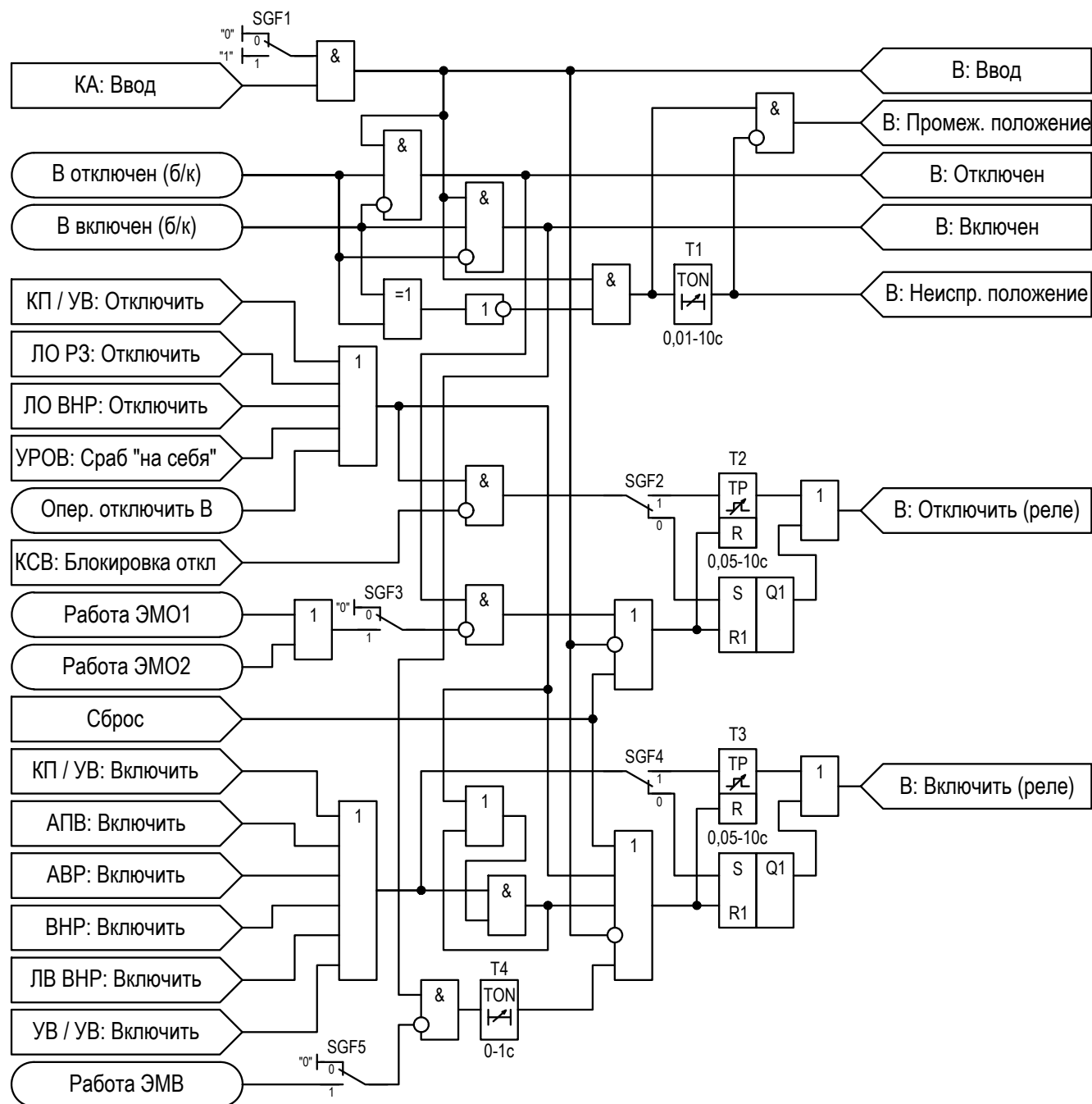
Рисунок 2.65 – Функциональная схема «Выключатель»
